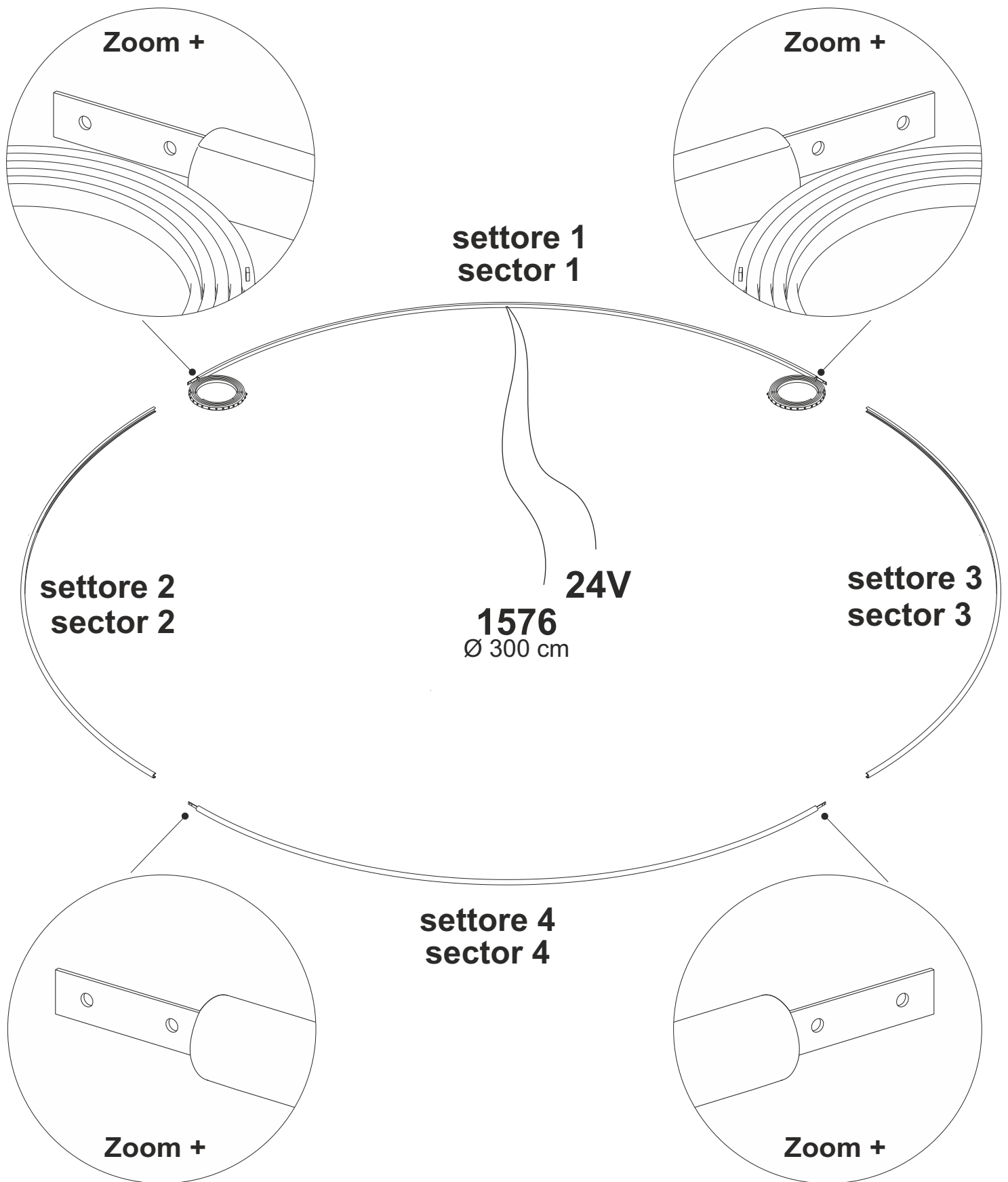
Assemblaggio dei 4 settori a terra Assembly of the 4 sectors on the ground
