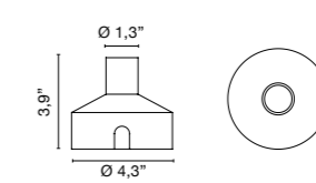
Draining box Encofrado drenante
