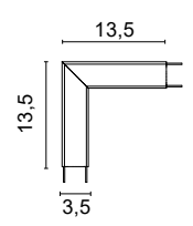
0941 Angolo 90° - 90°corner .01 Bianco - White
